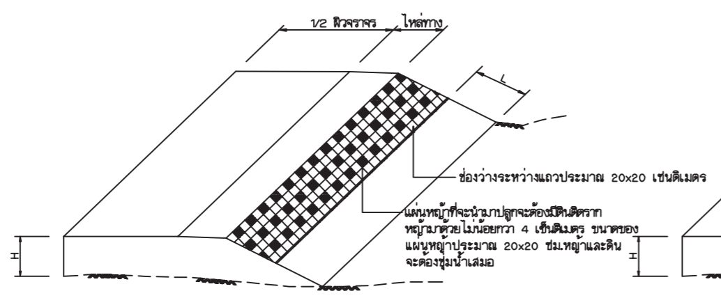
ภาพมิติแสดงการปลูกหญ้าแบบปักเป็นหย่อม (DOT SODDING)
