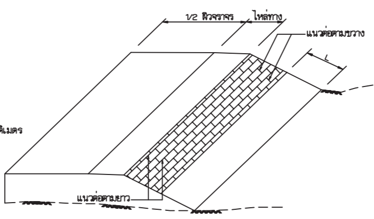
ภาพมิติแสดงการปลูกหญ้าแบบปูแผ่นเต็มพื้นที่ (BLOCK SODDING)
