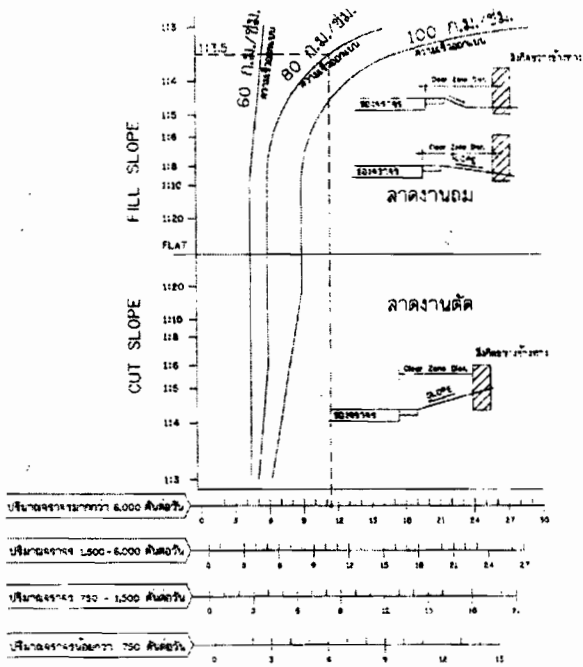
รูปที่ 1 ขนาดพื้นที่ทางวิ่งและเขตปลอดสิ่งกีดขวาง (Clear Zone Distance) เมตร Modified from Table 2.2 Roadside Design Guide, 2000
