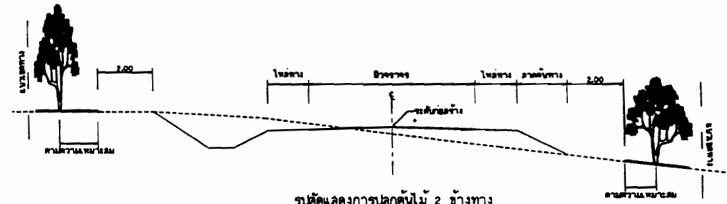
รูปตัดแสดงการปลูกต้นไม้ 2 ข้างทาง กรณีที่เป็นดินคันและดินถม
