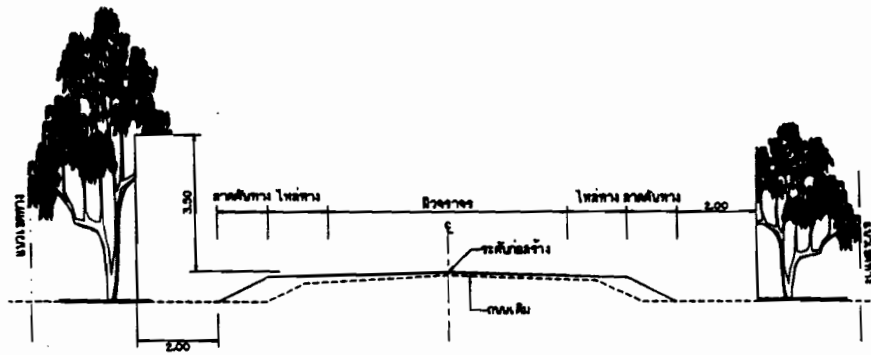
รูปตัดแสดงการบำรุงรักษาต้นไม้ 2 ข้างทาง
